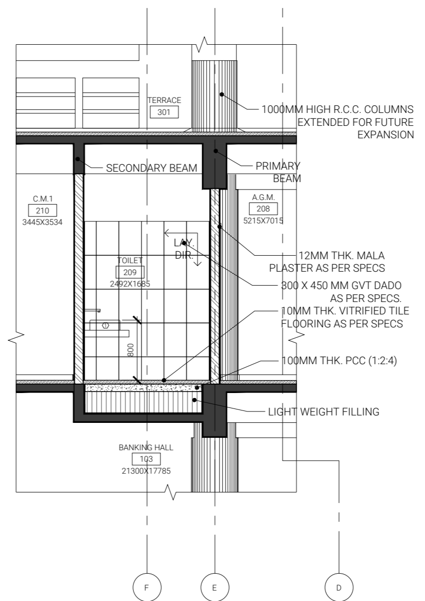
5 ELEVATION 2 1:50
