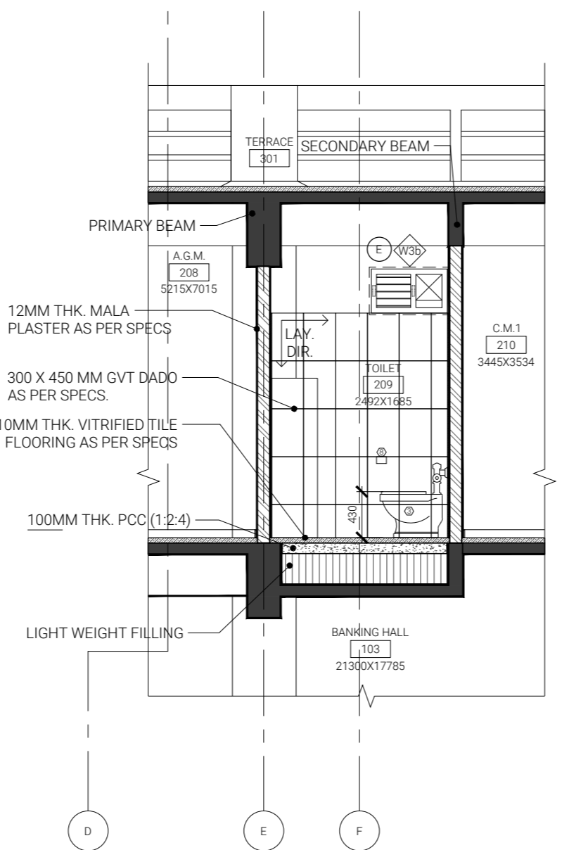
4 ELEVATION 4 1:50
