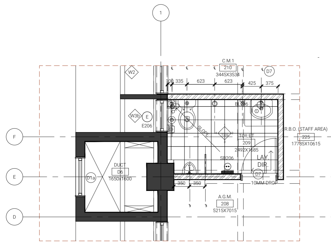
1 PLAN 1:50
